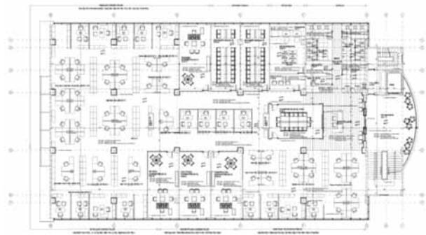
Birinci Kat Planı
